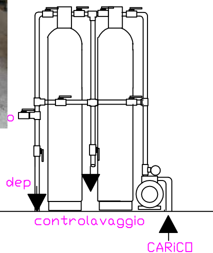
SCHEMA
