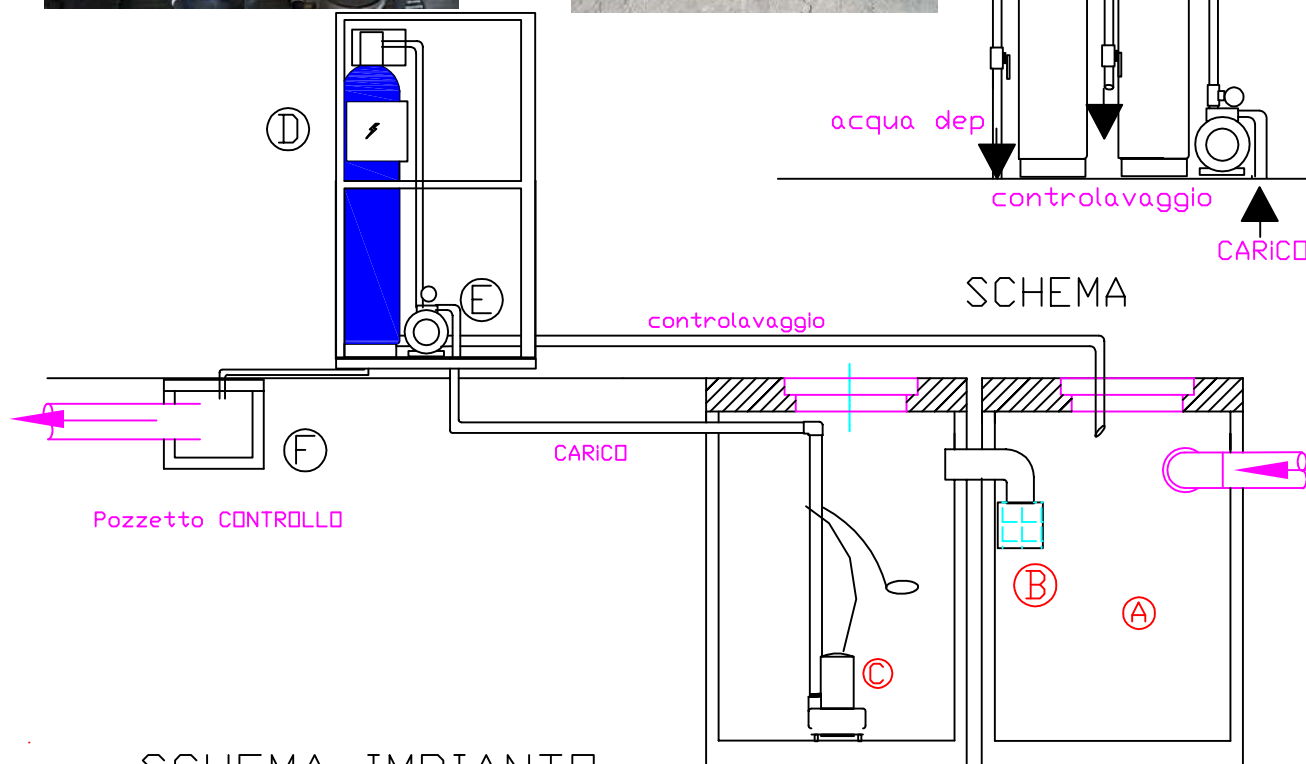
SCHEMA IMPIANTO
